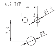
Leiterplatte 2-polig / PCB 2 poles
