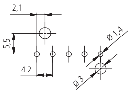
Empfehlung Lochbild Leiterplatte Recommendation of PCB holes
