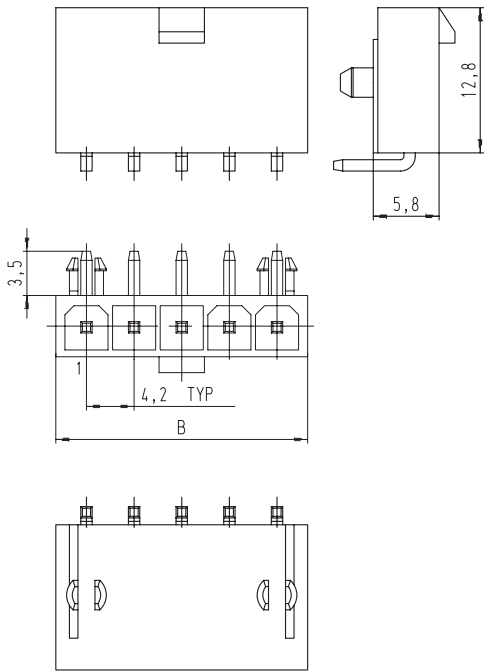
Beispiel Leiterplatte 5-polig / Sample PCB 5 poles
