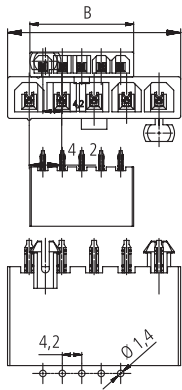
Empfehlung Lochbild Leiterplatte Recommendation of PCB holes
